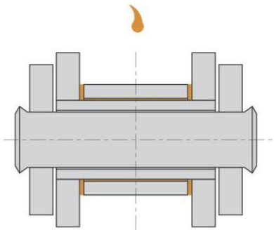
a) 错误的给油方式 Incorrect method
