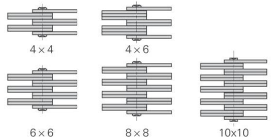
链板组合 Plate lacing
