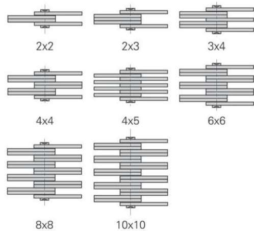
链板组合 Plate lacing
