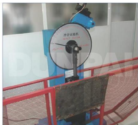
夏比缺口冲击试验机 Charpy Notch Impact test machine
