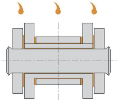
b) 正确的给油方式 Correct method
