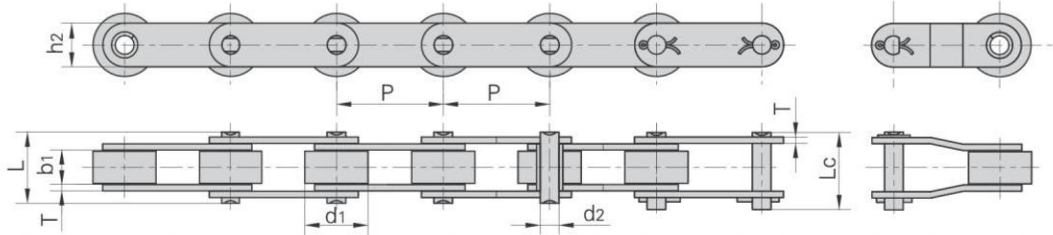
大滚子型 Large Roller Type
