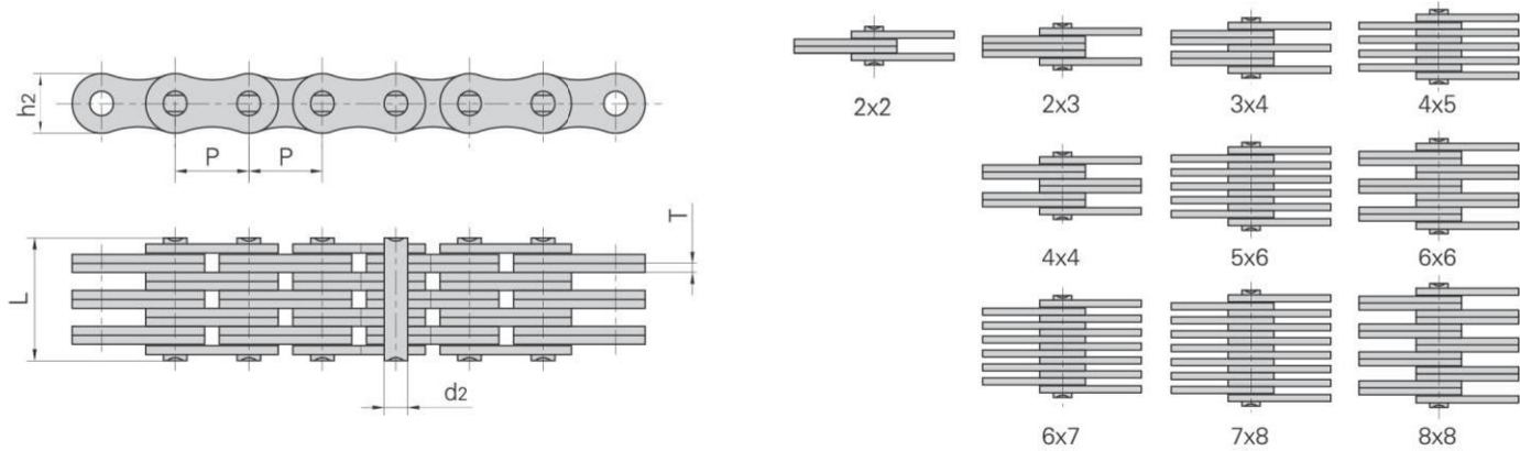
链板组合 Plate lacing
