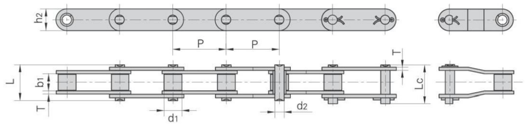
小滚子型 Small Roller Type
