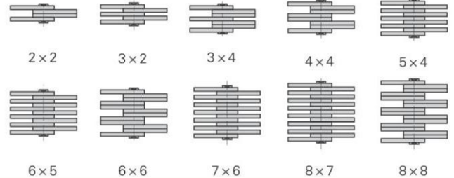
链板组合 Plate lacing
