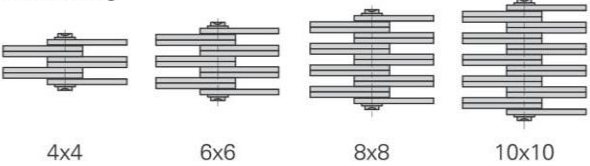
链板组合 Plate lacing
