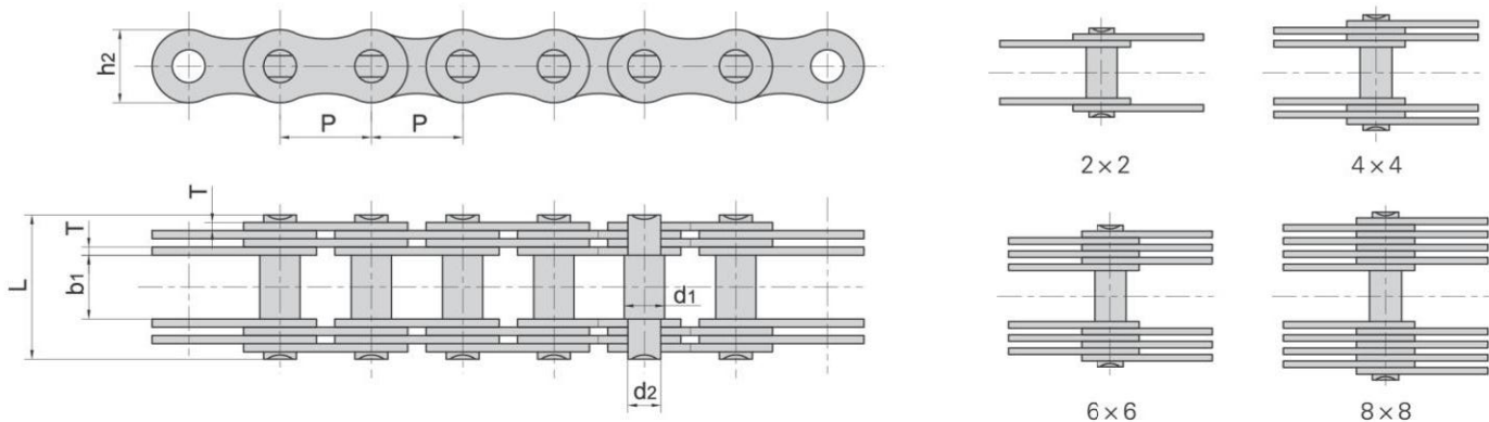
链板组合 Plate lacing
